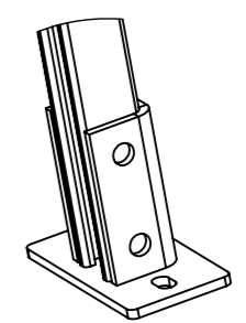
DÉTAIL C ECHELLE 1 : 5
